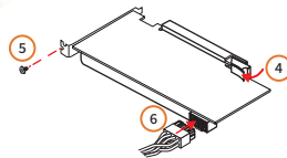
图2-10 显卡安装
