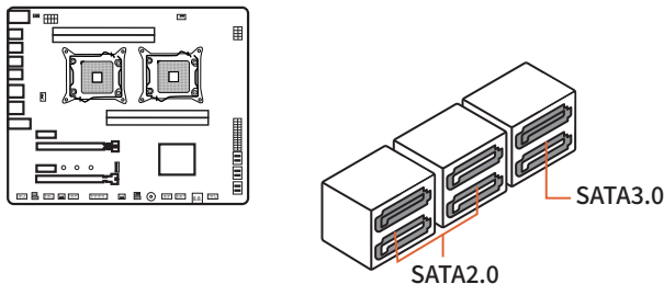
图2 -11 SATA接口
