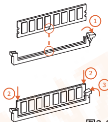
图2-9 内存安装
