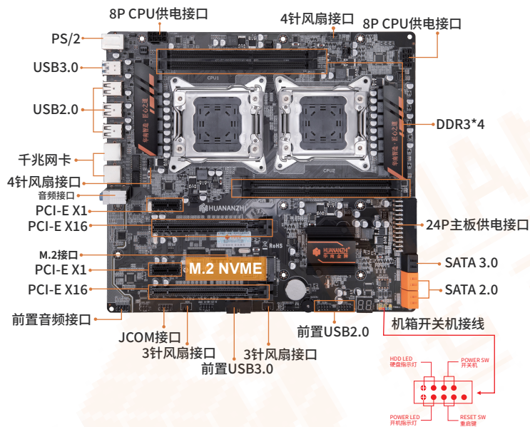
图1-1 X79-4D双路主板图解
